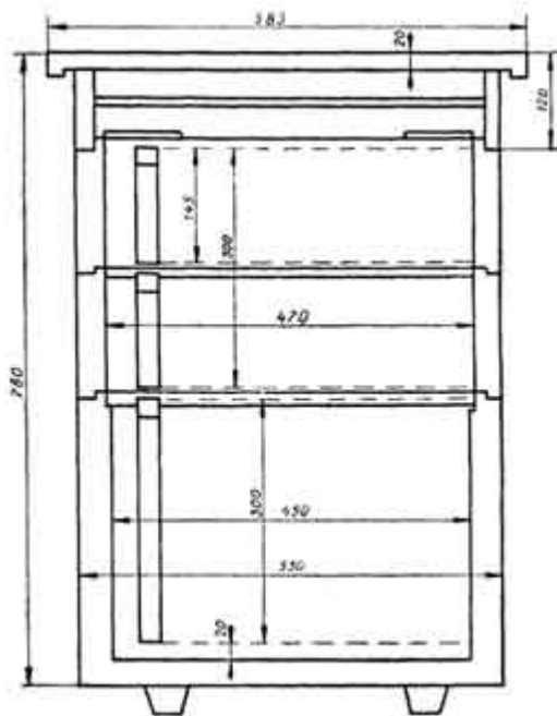
Поперечный разрез улья-стояка с двумя магазинами
