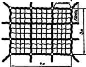
Строп-сетка с кольцами для увязки ульев на машине
